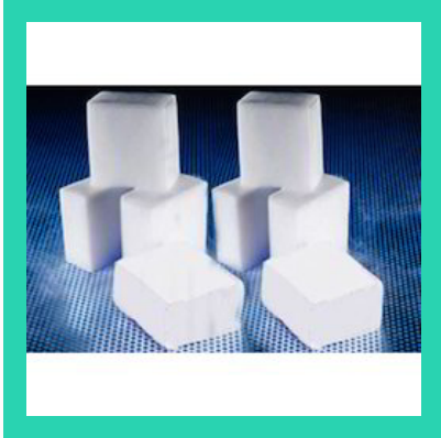
Solid Co2
